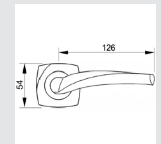
0R6853.000.** Door handle on roses
