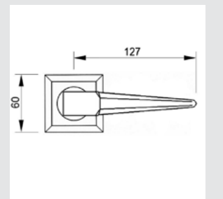
0R6454.000.** Door handle on roses
